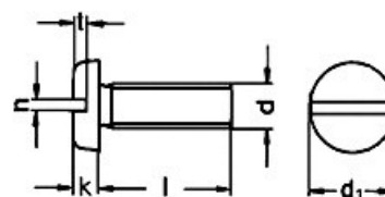
Βίδα με μεγάλο τραπεζοειδές κεφάλι, για ίσιο κατσαβίδι Slotted pan head screw
